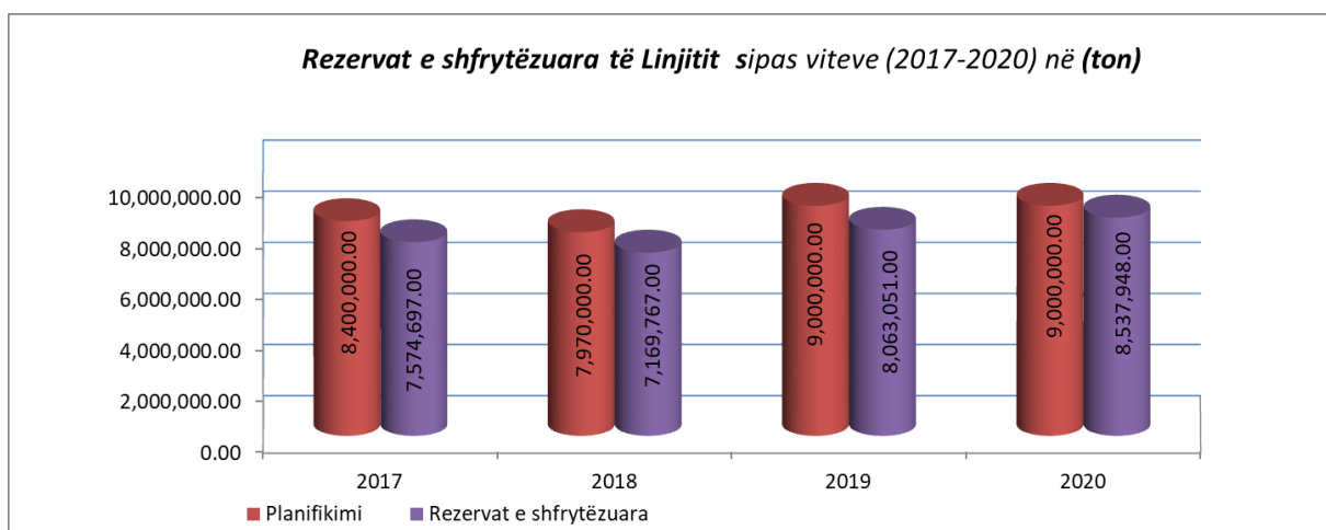
Figura 16. Diagrami i gjendjes së rezervave të shfrytëzuara - mineralet energjetike-Linjitit, 2017-2020
