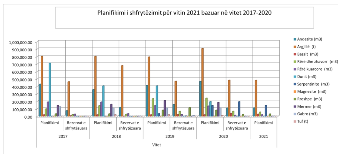
Figura 25. Diagrami i planifikimit të shfrytëzimit të rezervave minerale jo-metalore për vitin 2021 bazuar në vitet 2017-2020
