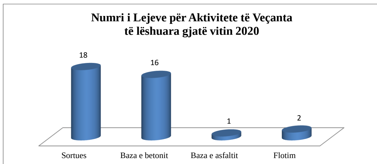
Figura 14. Grafiku i lejeve të lëshuara për vitin 2020 për aktivitete të veçanta.
