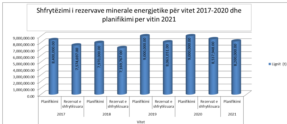
Figura 23. Planifikimi i shfrytëzimit të rezervave minerale energjetike (linjtit) për vitin 2021 bazuar në vitet 2017-2020
