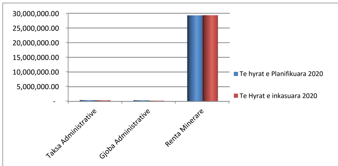
Figura 40. Planifikimi dhe inkasimi i të hyrave për vitin 2020
