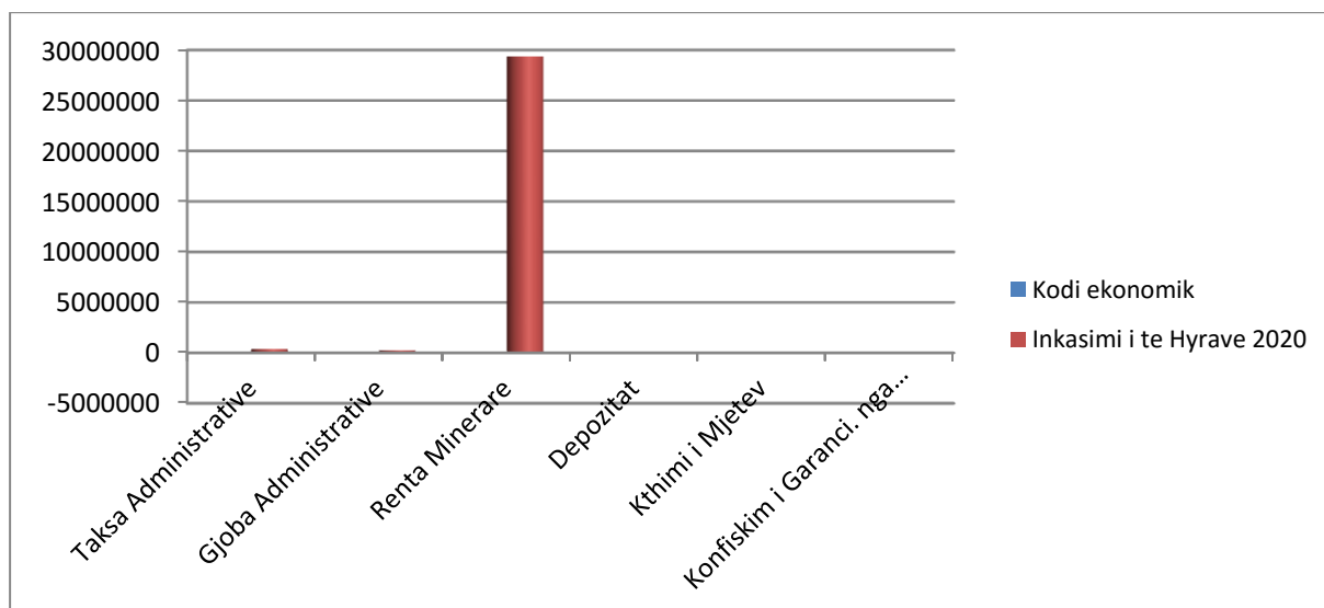
Figura 39. Inkasimi i të hyrave për vitin 2020
