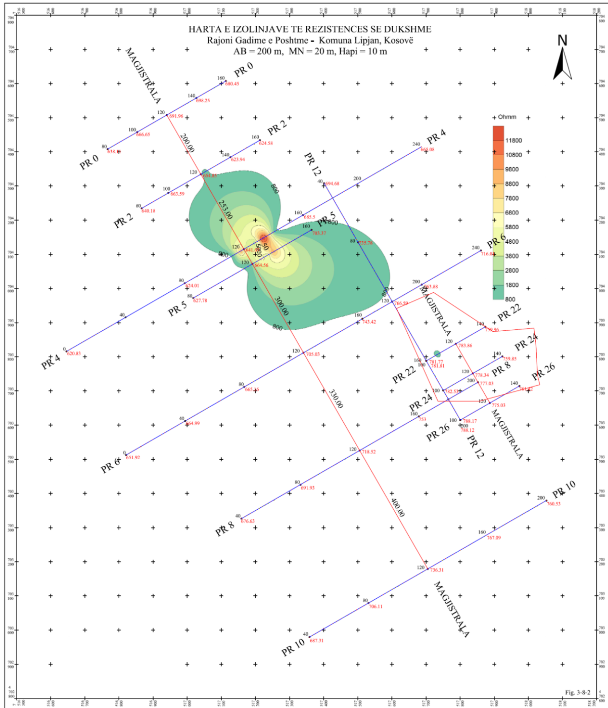
Figura 45. Karta prividne optpornosti izolinja
