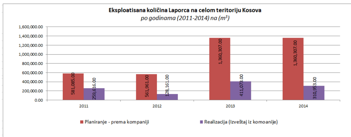
Figura 28. Grafički prikaz korišćene količine mergele u celoj teritoriji Kosova, u vremenskom periodu 2011-2014
