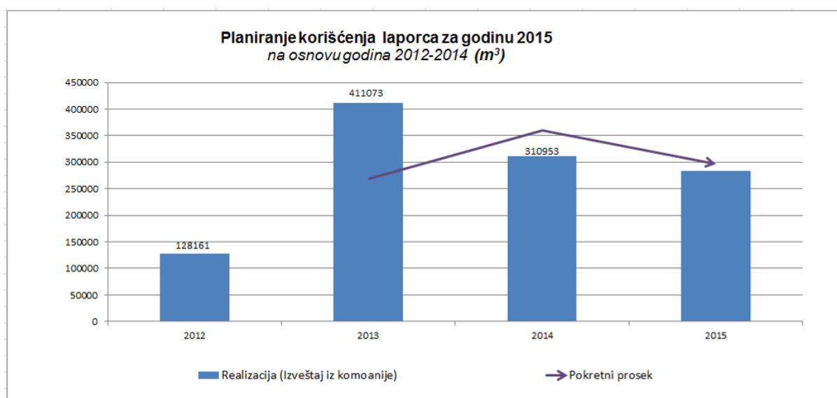
Figura 29. Prikaz proizvodnje mergele i pokretni prosekok, na osnovu proizvodnje od 2012-2014
