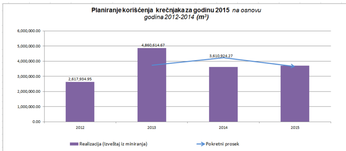
Figura 19. Pregled proizvodnje krečnjaka i pokretni prosek, na osnovu proizvodnje od 2012-2014
