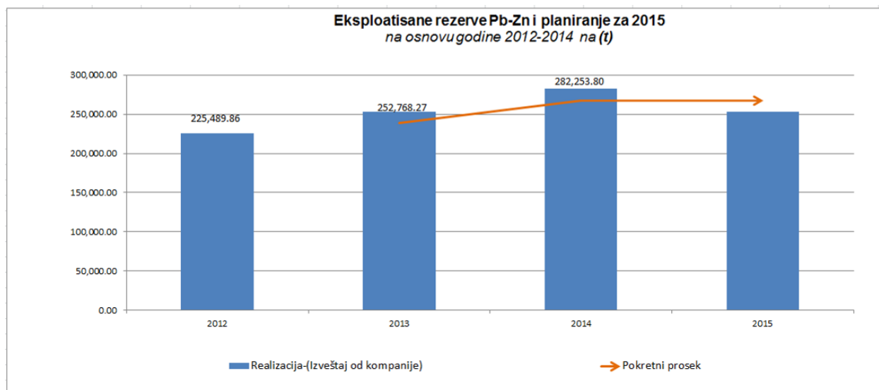
Figura 34. Prikaz proizvodnje Pb-Zn i pokretni prosek, na osnovu proizvodnje od 2012-2014
