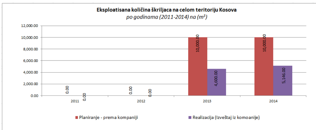
Figura 30. Grafički prikaz korišćene količine škriljca u celoj teritoriji Kosova, u vremenskom periodu 2011-2014
