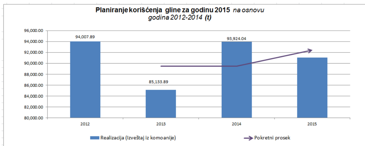
Figura 17. Prikaz proizvodnje gline i pokretni prosek, na osnovu proizvodnje od 2012-2014
