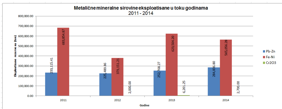
Figura 40. Korišćene rezerve u metalnim depozitima tokom preioda 2011-2014
