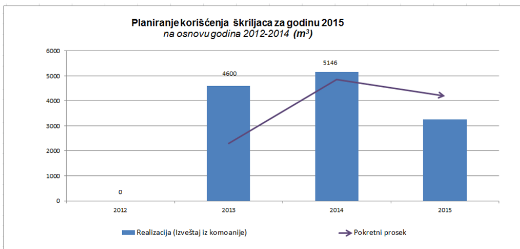
Figura 31. Prikaz proizvodnje škriljca i pokretni prosek, na osnovu proizvodnje od 2012-2014
