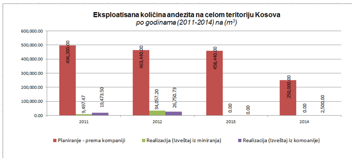
Figura 14. Prikazanje korišćene količine andezita u celoj teritoriji Kosova, u vremenskom periodu od 2011-2014
