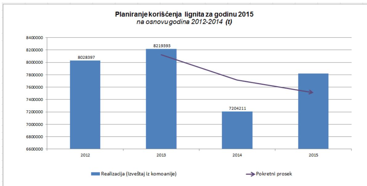
Figura 13. Pregled proizvodnje Lignita i pokretni prosek, to na osnovu proizvodnje od 2012-2014
