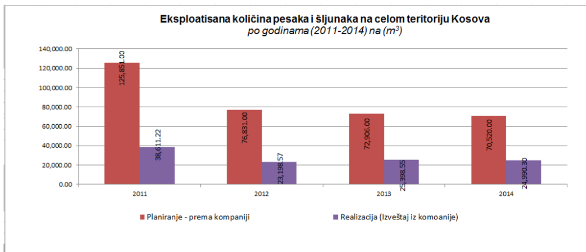
Figura 22. Grafički prikaz korišćene količine peska i šljunka u celoj teritoriji Kosova, u vremenskom periodu 2011-2014
