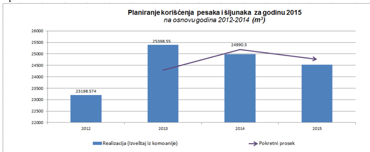
Figura 23. Prikaz proizvodnje peska-šljunka i pokretni prosek, na osnovu proizvodnje od 2012-2014
