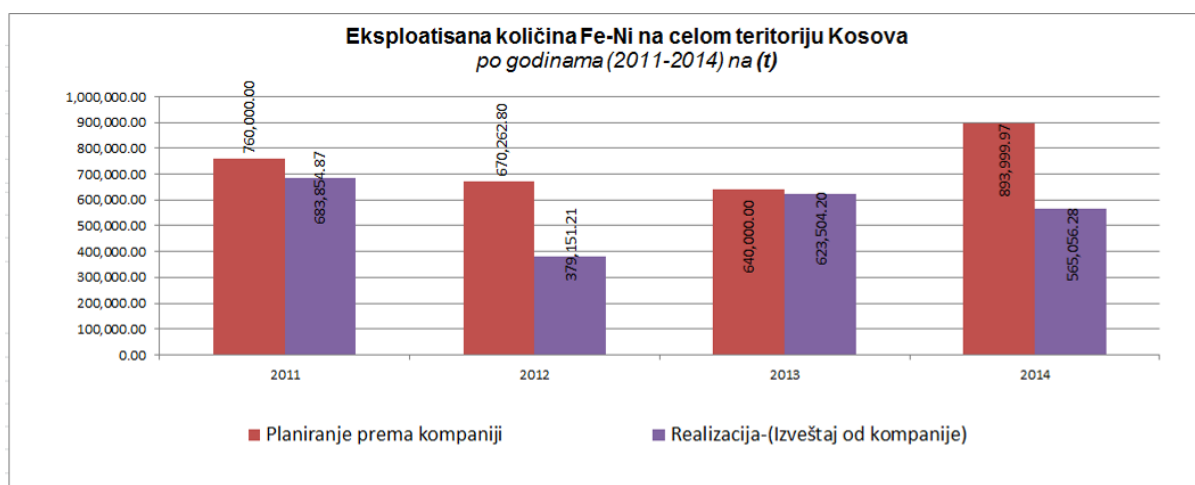
Figura 36. Grafički prikaz korišćene količine Fe-Ni rude u celoj teritoriji Kosova, u vremenskom periodu 2011-2014
