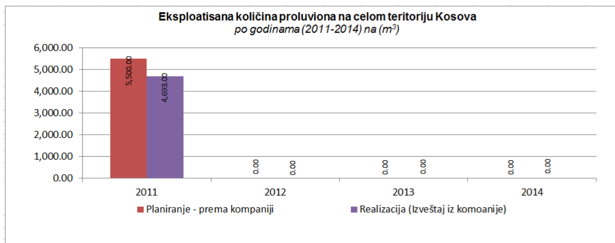
Figura 32. Grafički prikaz količine korišćenih proluviona u celoj teritoriji Kosova, u vremenskom periodu 2011-2014
