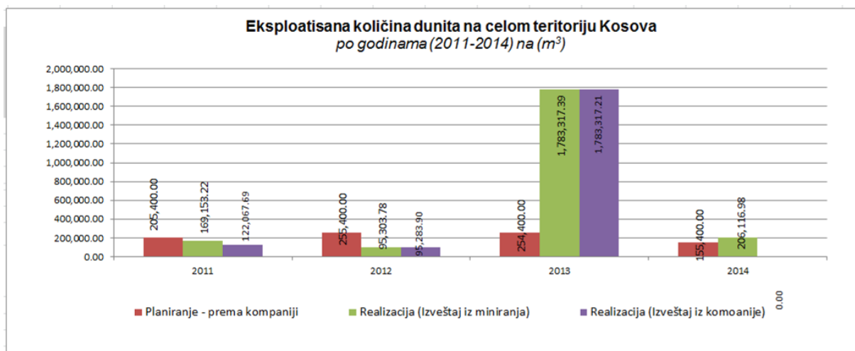
Figura 26. Grafički prikaz korišćene količine dunita u celoj teritoriji Kosova, u vremenskom periodu 2011-2014
