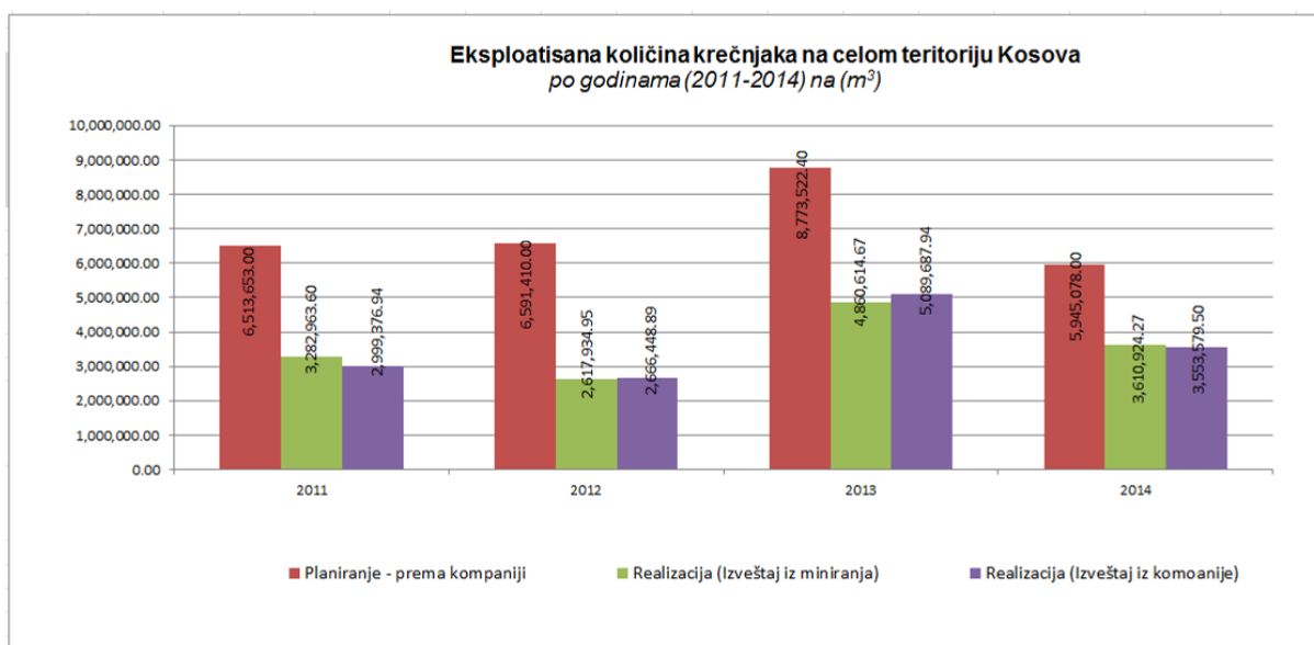
Figura 18. Grafički prikaz korišćene količine krečnjaka u celoj teritoriji Kosova, u vremenskom periodu 2011-2014
