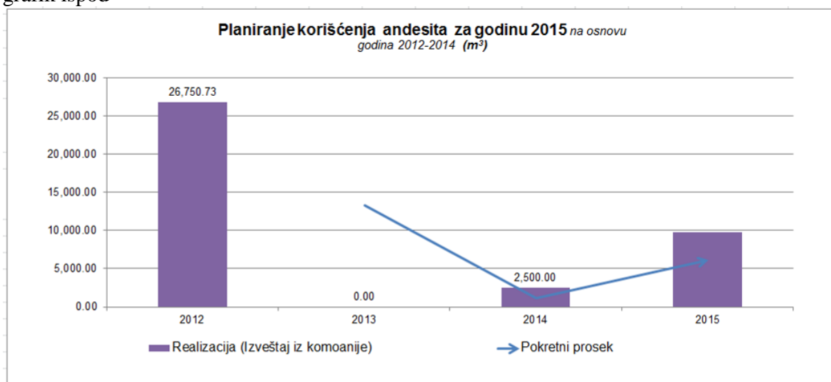
Figura 15. Pregled proizvodnje andezita i pokretni prosek, to na osnovu proizvodnje od 2012-2014
