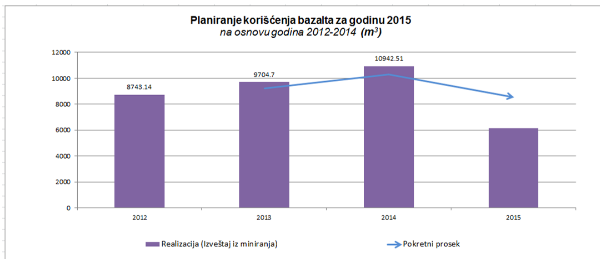
Figura 21. Pregled proizvodnje bazalta i pokretni prosek, na osnovu proizvodnje od 2012-2014
