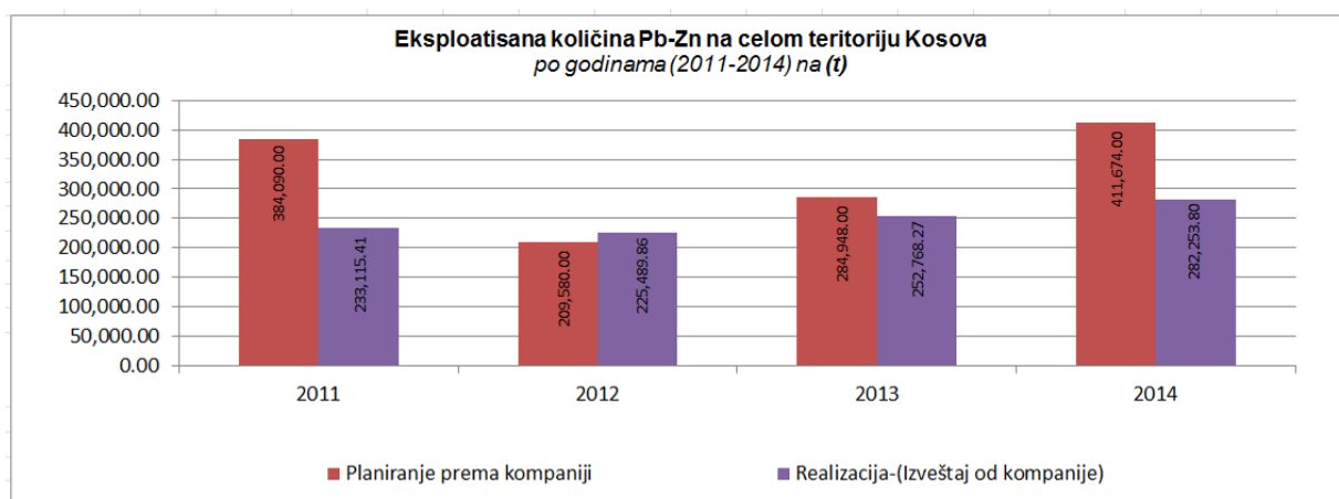
Figura 33. Grafički prikaz korišćene količine rude Pb-Zn u celoj teritoriji Kosova, u vremnskom periodu 2011-2014
