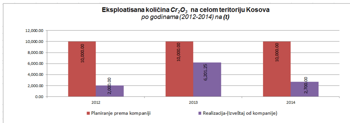
Figura 38. Grafički prikaz korišćene količine Cr_2O_3 rude u celoj teritoriji Kosova, u vremenskom periodu 2012-2014
