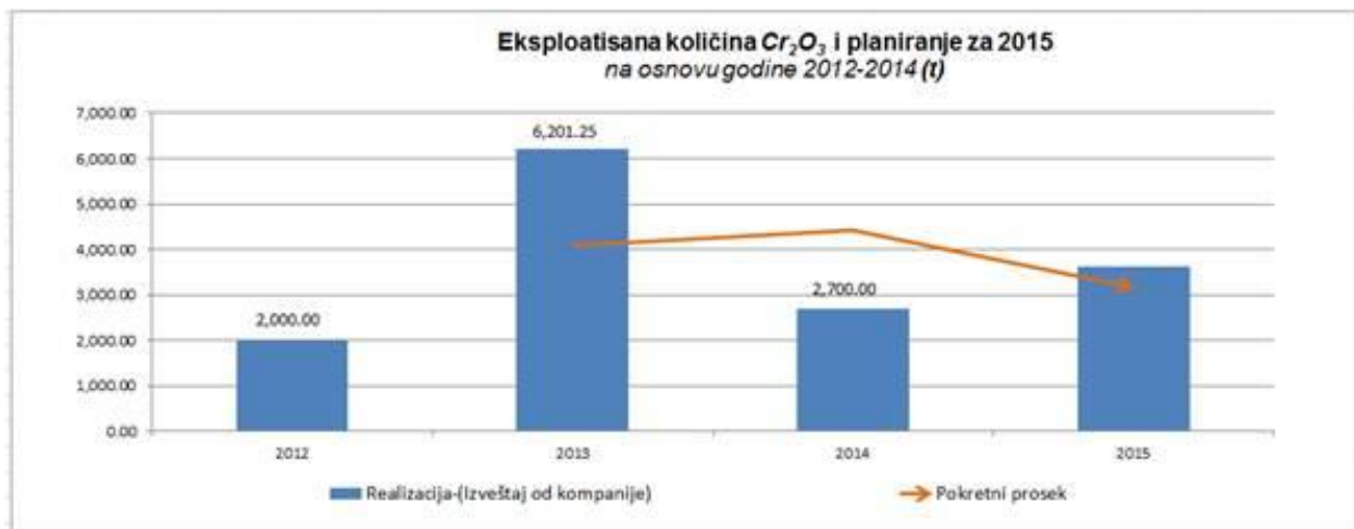
Figura 39. Pregled proizvodnje Cr 2 O 3 i pokretni prosek, to baziran na proizvodnji od 2012-2014
