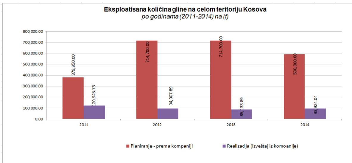
Figura 16. Tabela prikaz korišćene količine gline u celoj teritoriji Kosova, u vremenskom periodu 2011-2014
