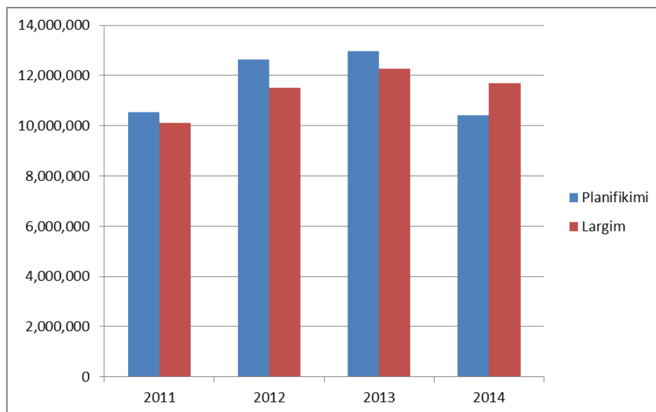
Figura 45. Planiranje-proizvodnja uklanjanja pustoši period 2011-2014
