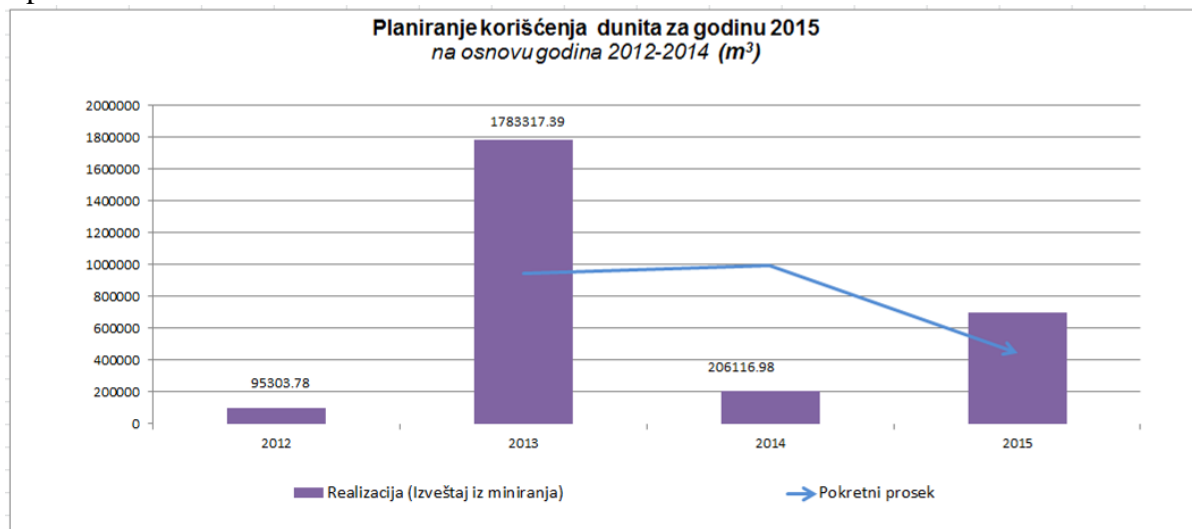
Figura 27. Prikaz proizvodnje dunita i pokretni prosek, na osnovu proizvodnje od 2012-2014
