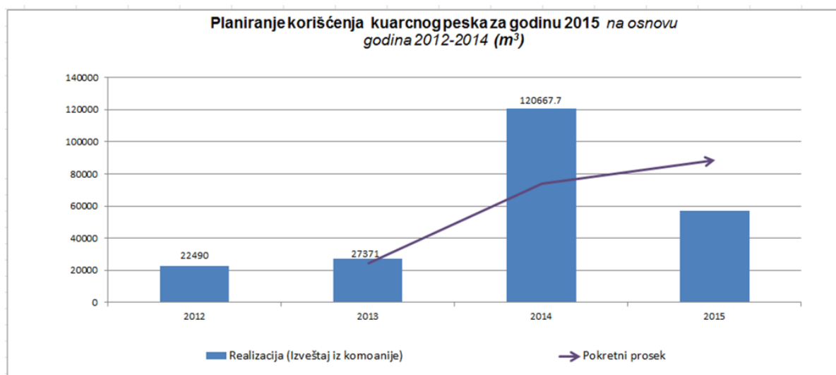
Figura 25. Prikaz proizvodnje kvarcnog peska i pokretni prosek, na osnovu proizvodnje od 2012-2014
