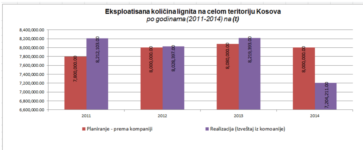
Figura 12. Grafički prikaz količine korišćenog lignita u celoj teritoriji Kosova, u vremenskom periodu 2011-2014
