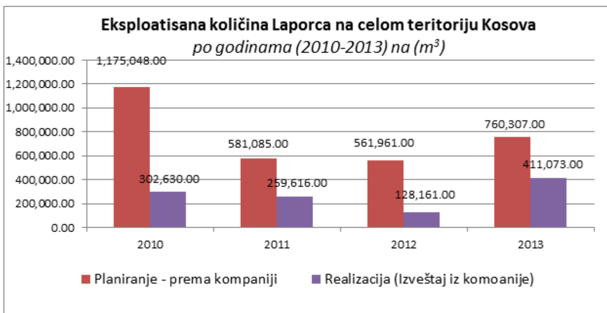
Figura 21. Korišćena količina laporca u teritoriji Kosova, u periodu od 2010-2013
