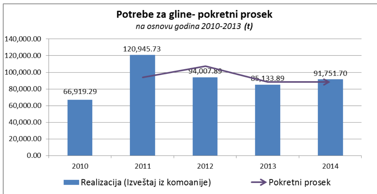
Figura 10. Proizvodnja (Pokretni prosek) gline ona se zasniva na proizvodnji od 2010-2013
