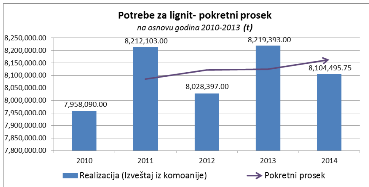
Figura 6. Proizvodnja (Pokretni prosek) lignita ona se zasniva na proizvodnji od 2010-2013
