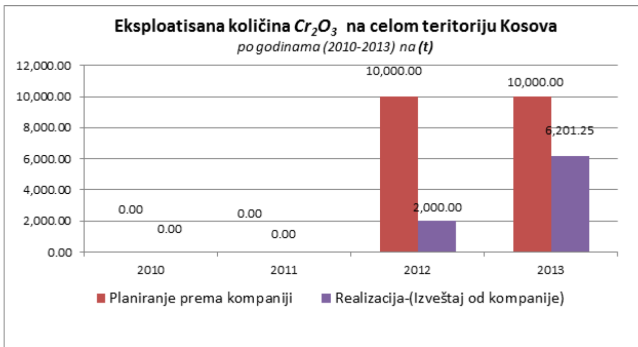
Figura 31. Korišćena količina rude \text{Cr}_2\text{O}_3 u teritoriji Kosova, u periodu od 2010-2013
