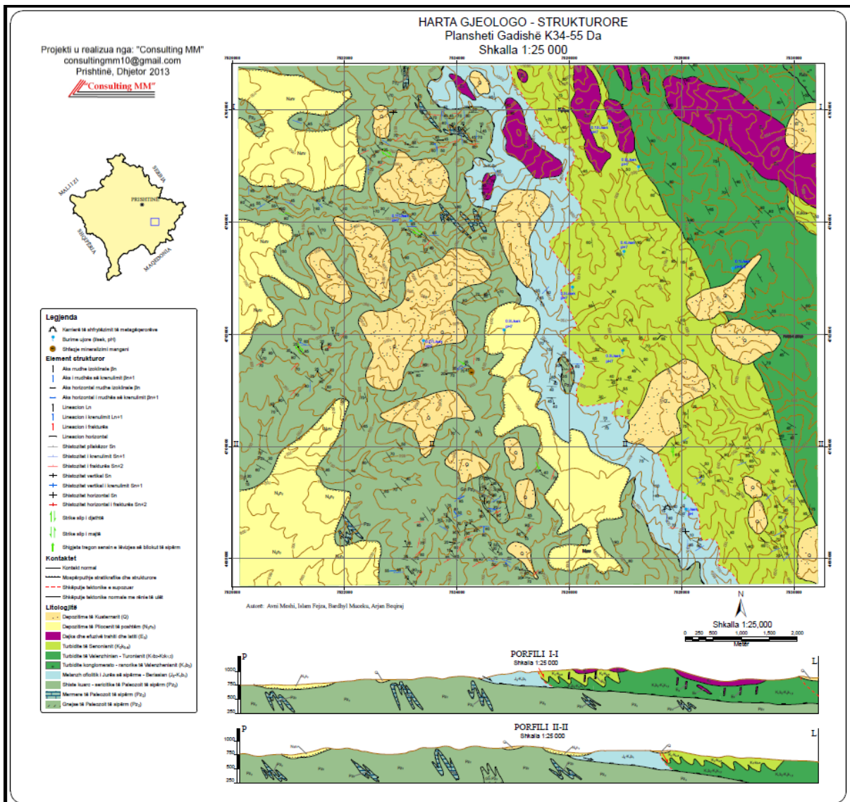
Figura 33. Geološka mapa Planšiete Gadiša K34-55 Da na stepenu 1 : 25 000
