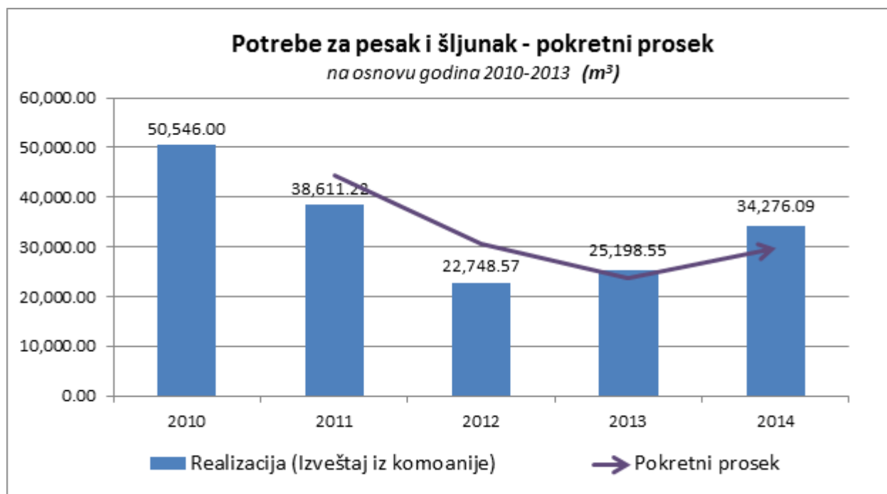
Figura 16. Proizvodnja (Pokretni prosek) peska i šljunka ona se zasniva na proizvodnji od 2010-2013
