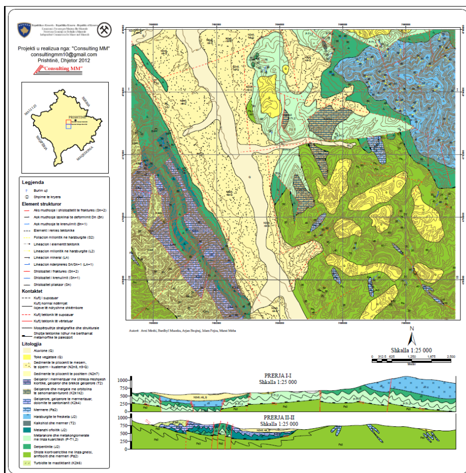
Figura 5. Geološka mapa Planchietta Blinaja na stepenu 1:25 000
