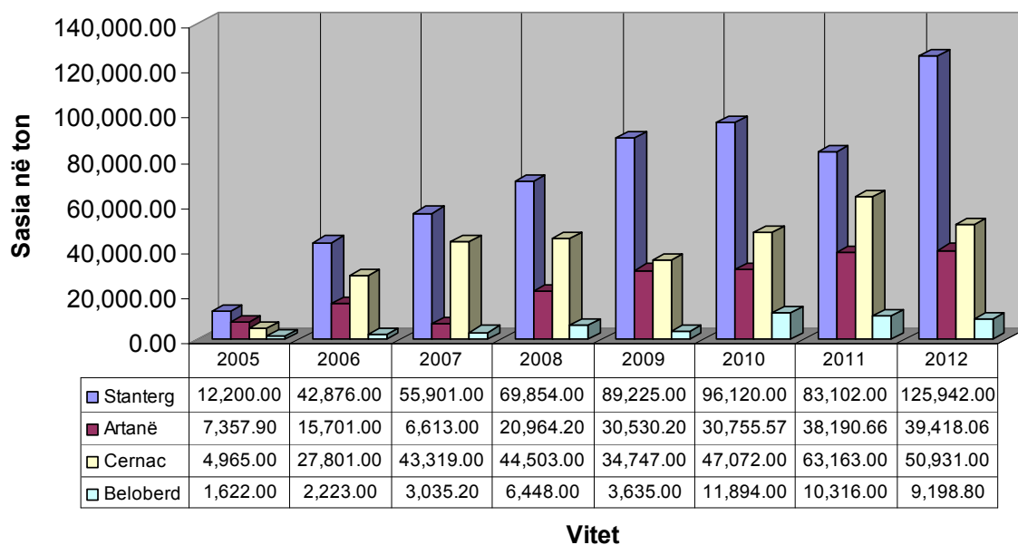
Figura 12. Proizvodnja Pb-Zn prema kompanijama i godinama
