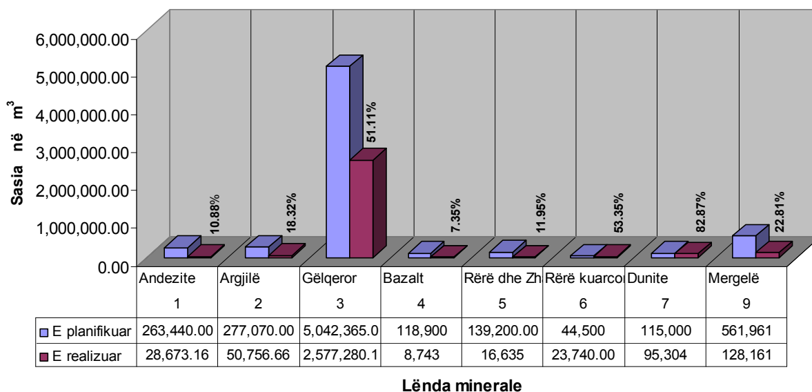
Figura 7. Korišćenje rezerve mineralnih građevinskih sirovina
