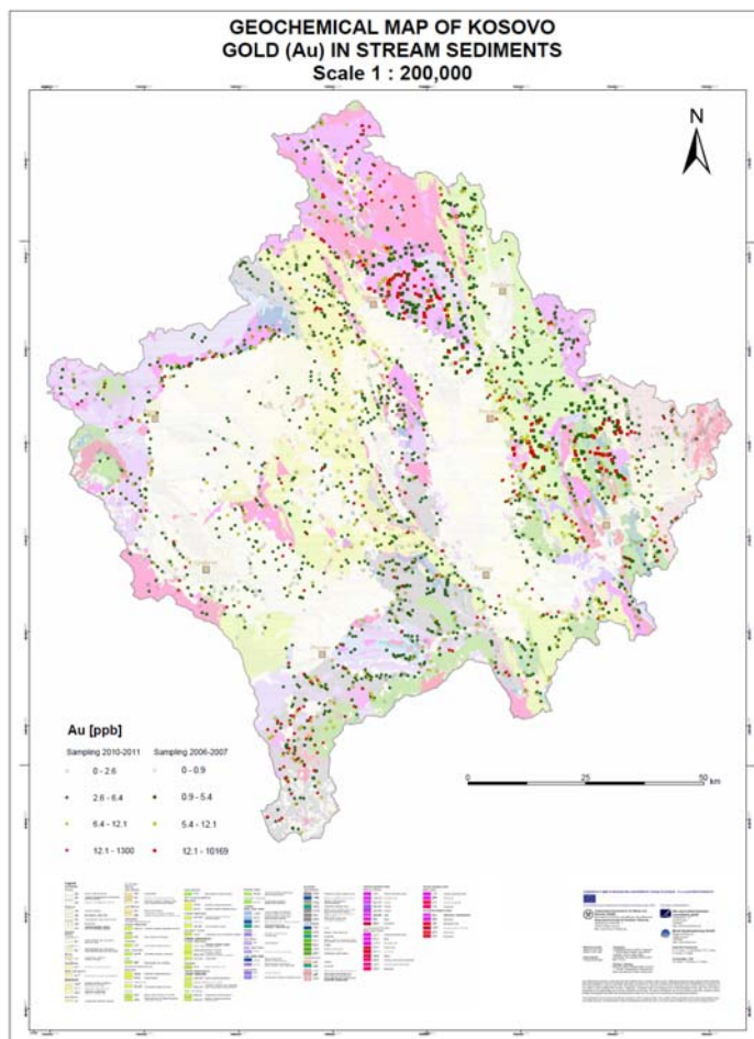
Figura 6. Distribucija mineralizacije zlata u teritoriji Kosova.
