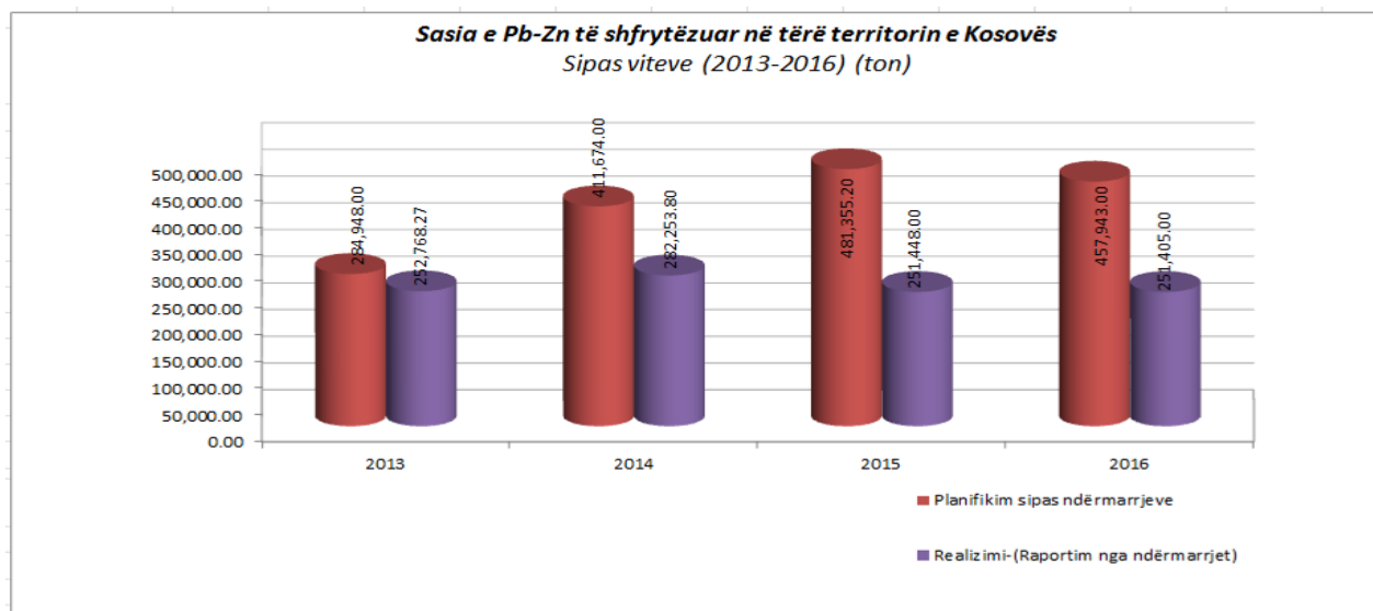
Figura 16. Paraqitje në grafik e sasisë së shfrytëzuar të xehes së Pb-Zn në tërë territorin e Kosovës, në periudhën kohore 2013-2016.
