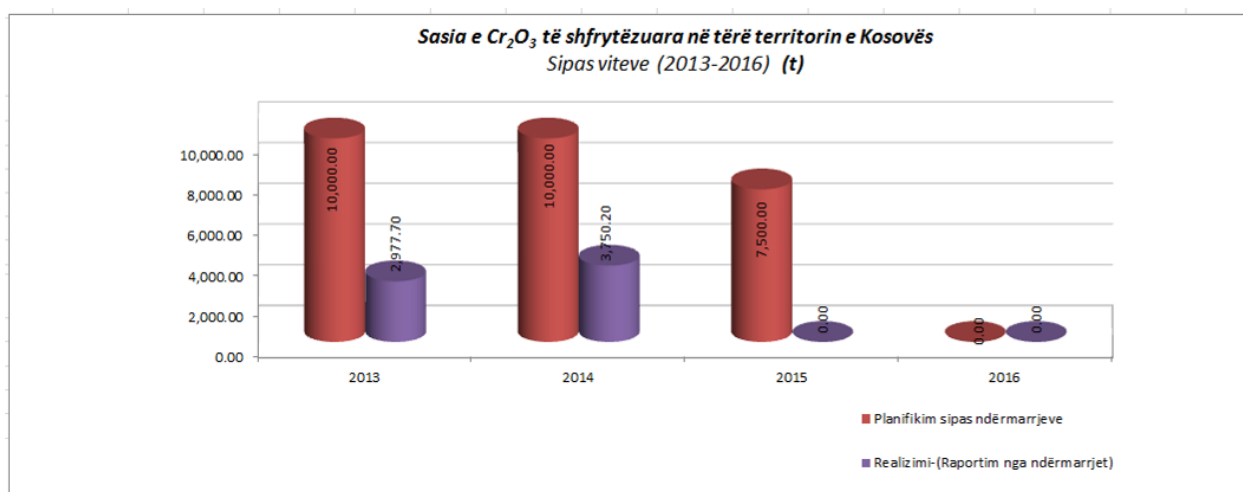
Figura 18. Paraqitje në grafik e sasisë së shfrytëzuar të xehes së \text{Cr}_2\text{O}_3 në tërë territorin e Kosovës, në periudhën kohore 2013-2016
