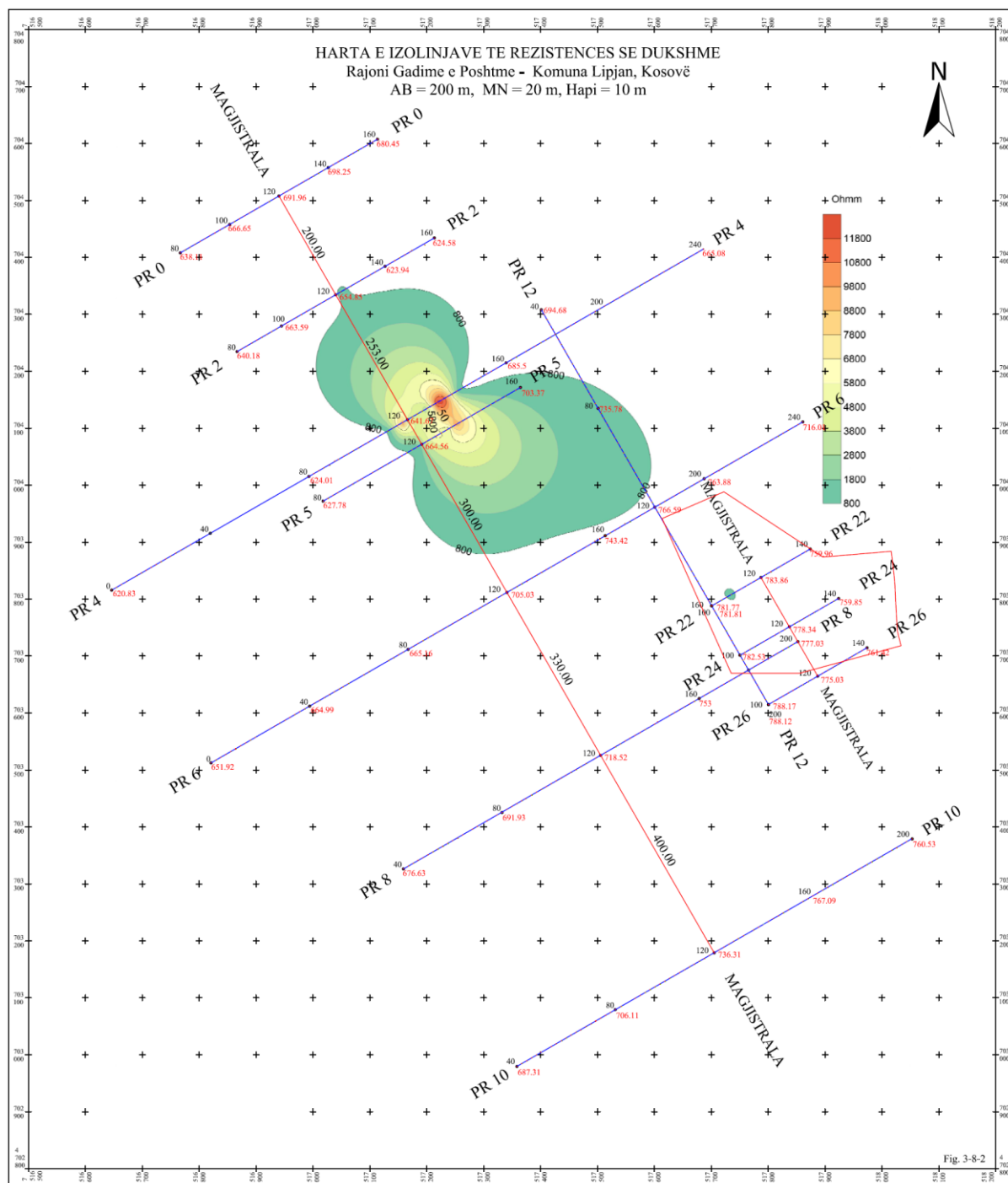
Figura 45. Harta e izolinjave të rezistencës së dukshme
