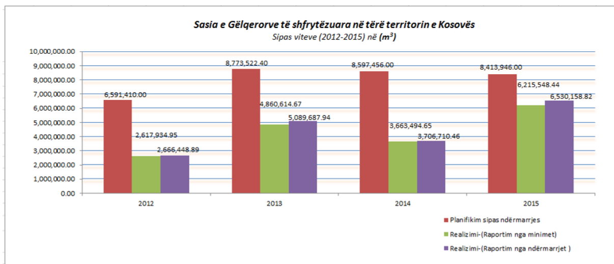
Figura 26. Paraqitje në grafik e sasisë së shfrytëzuar të gëlqerorëve në tërë territorin e Kosovës, e bazuar kjo në prodhimitarinë nga 2012-2015
