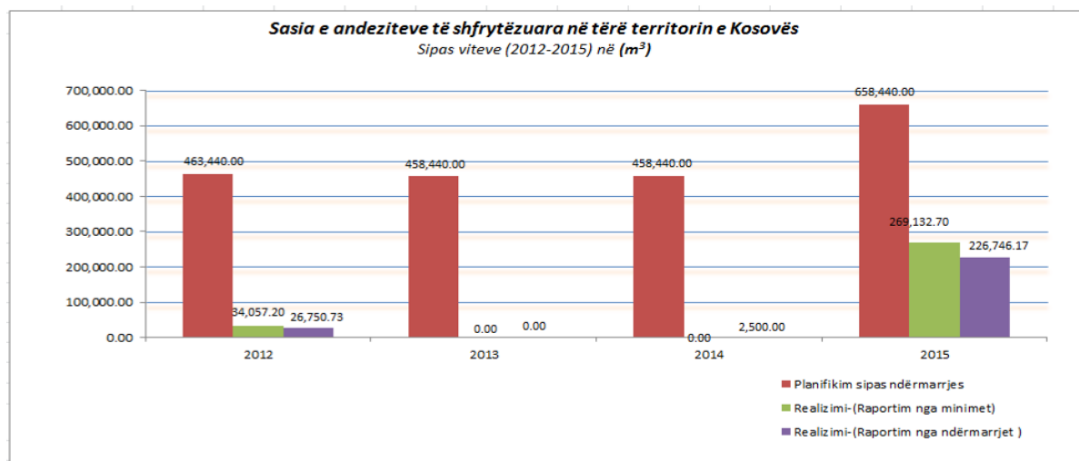
Figura 22. Paraqitje e sasisë së shfrytëzuar të andeziteve në tërë territorin e Kosovës, në periudhën kohore 2012-2015
