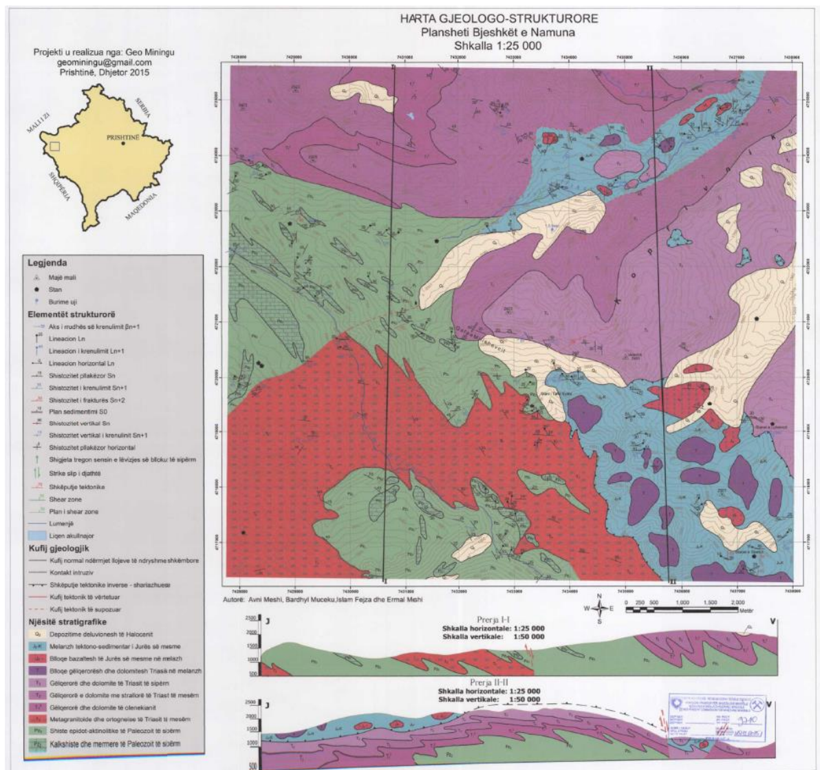
Figura 40. Harta gjeologjike e Planshetit Krasmiroc-K34-53 Ab në shkallë 1:25 000
