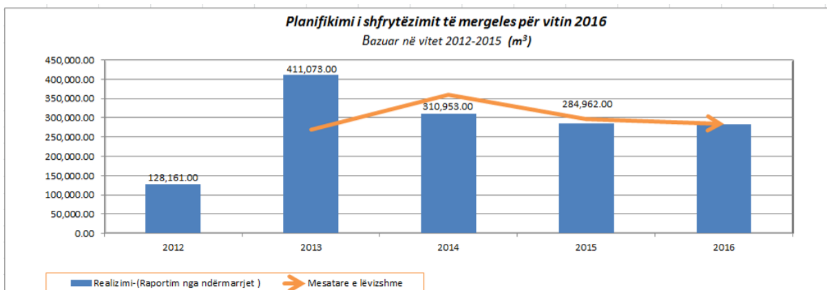
Figura 37. Paraqitje e prodhimtarisë së mergelës dhe mesatarja e lëvizshme, e bazuar kjo në prodhimtarinë nga 2012-2015
