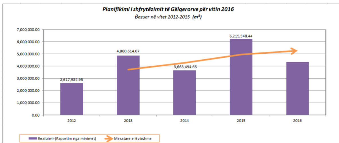
Figura 27. Paraqitje e prodhimit të gëlqerorëve dhe mesatarja e lëvizshme, e bazuar kjo në prodhimtarinë nga 2012-2015
