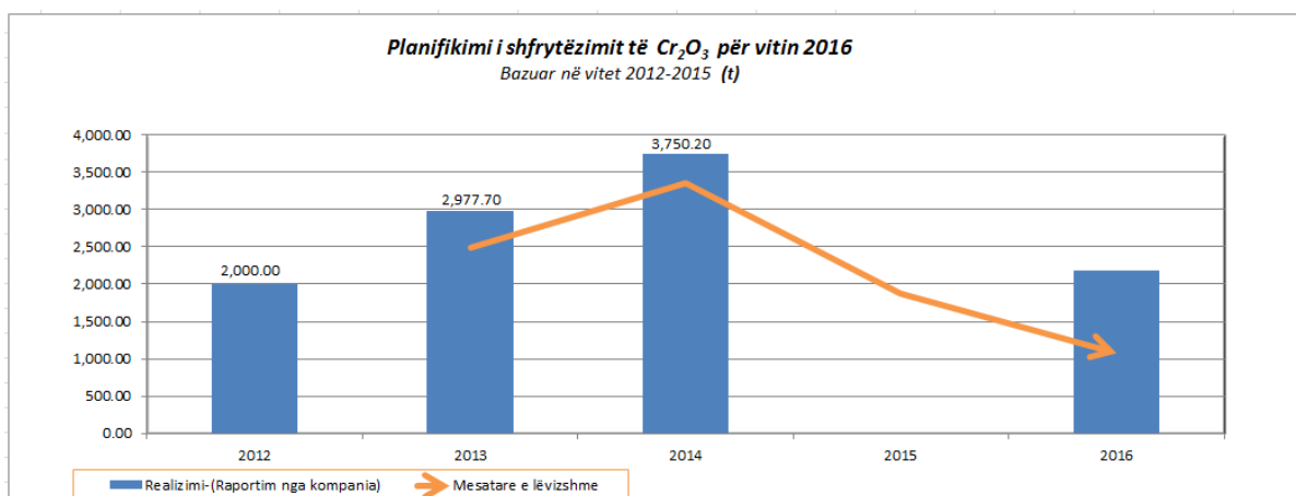
Figura 17. Paraqitje e prodhimitarisë së \text{Cr}_2\text{O}_3 dhe mesatarja e lëvizshme, e bazuar kjo në prodhimitarinë nga 2012-2015
