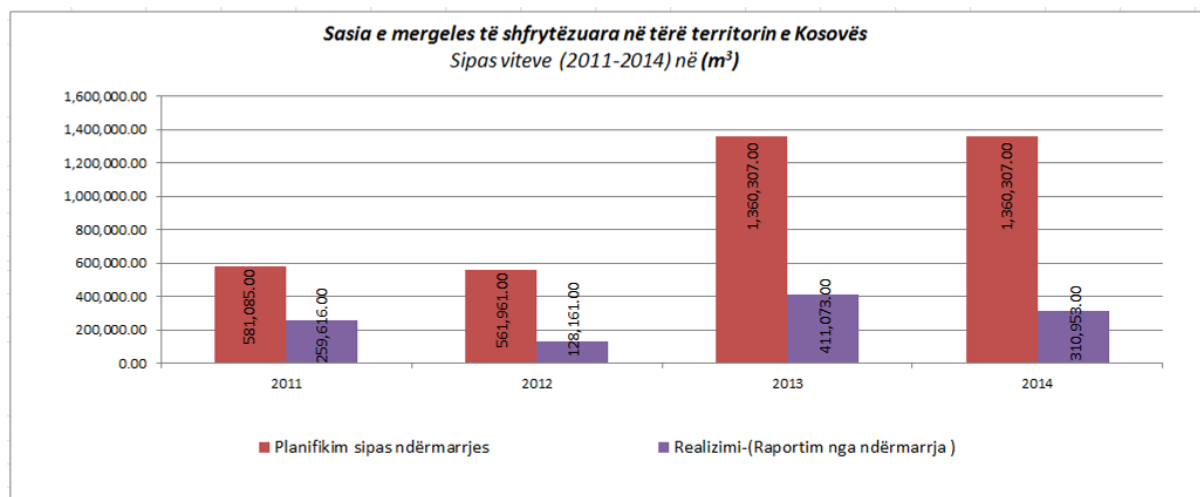
Figura 28. Paraqitje në grafik e sasisë së shfrytëzuar të mergelës në tërë territorin e Kosovës, në periudhën kohore 2011-2014
