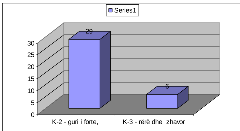
Figura 9. Numri i licencave për shfrytëzim sipas llojeve të lëndëve minerale
