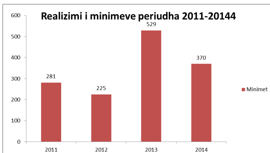
Figura 48. Realizimi i minimeve sipërfaqësore periudha 2011-2014
