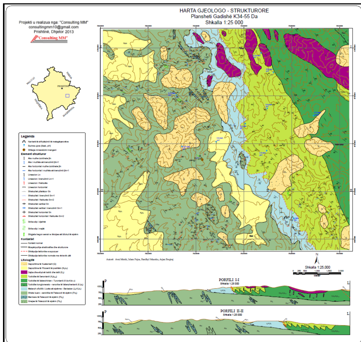
Figura 33. Harta gjeologjike e Planshetit Gadishë K34-55 Da në shkallë 1 : 25 000
