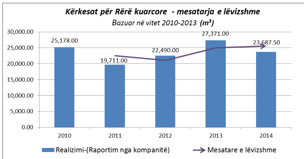
Figura 18. Prodhimtaria (mesatarja e lëvizshme) e rërës kuarcore e bazuar në prodhimtarinë 2010-2013
