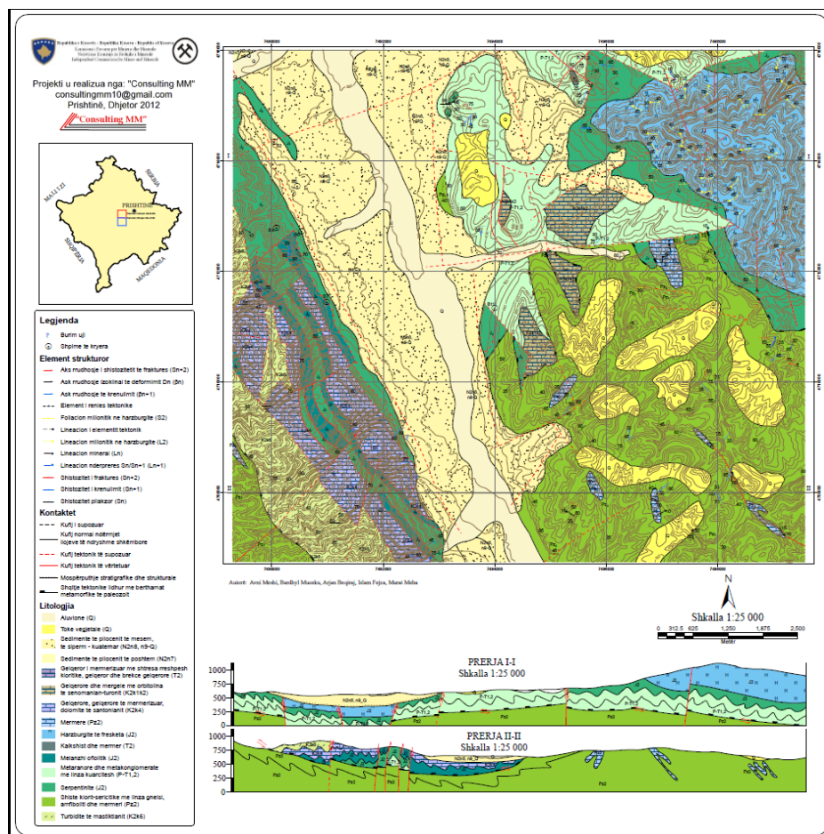
Figura 5. Harta gjeologjike e Planshetit të Blinajës në shkallë 1:25 000
