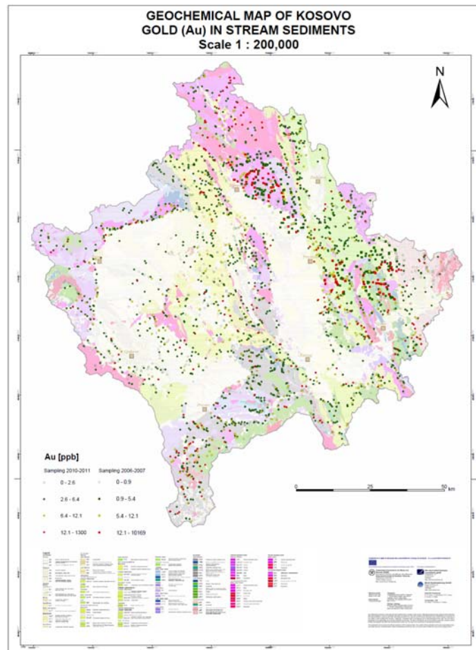
Figura 6. Shpërndarja e mineralizimeve të arit në territorin e Kosovës.
