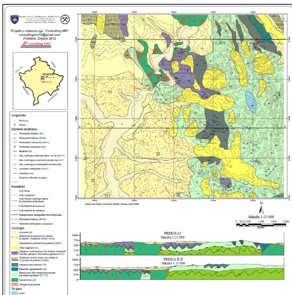
Figura 4. Harta gjeologjike e Planshetit të Drenasit në shkallë 1:25 000
