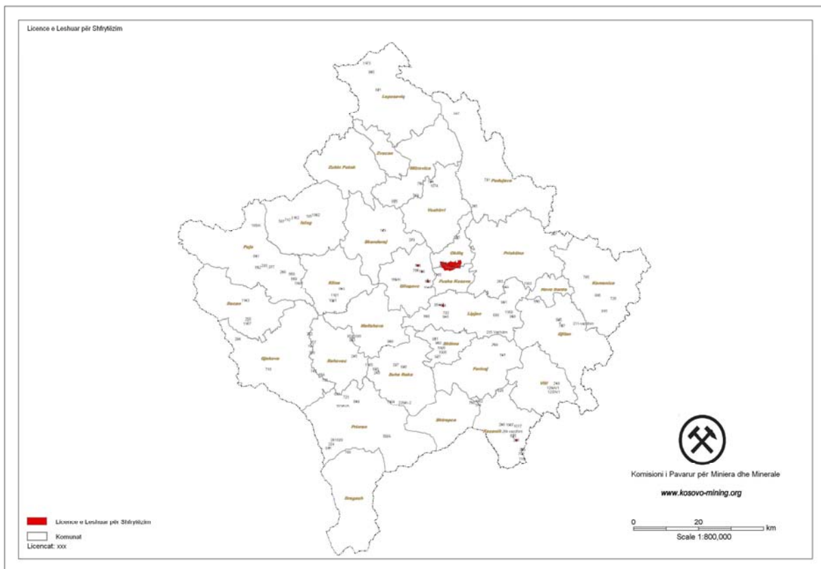
Figura 7. Harta e licencave të shfrytëzimit
