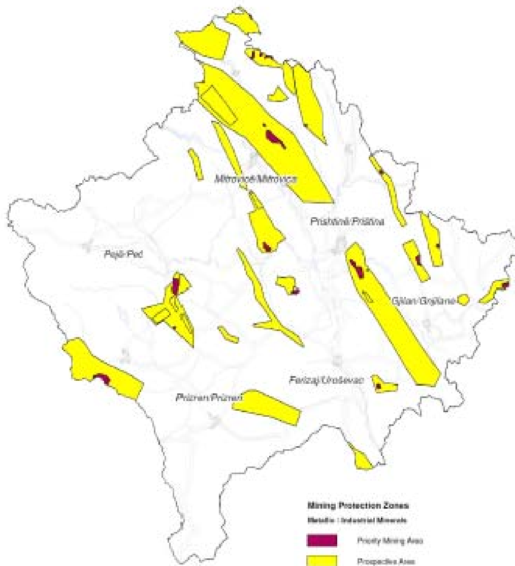
Figura 23. Hartë vështruese e Zonave të mbrojtura minerare të mineraleve metalike dhe industriale
