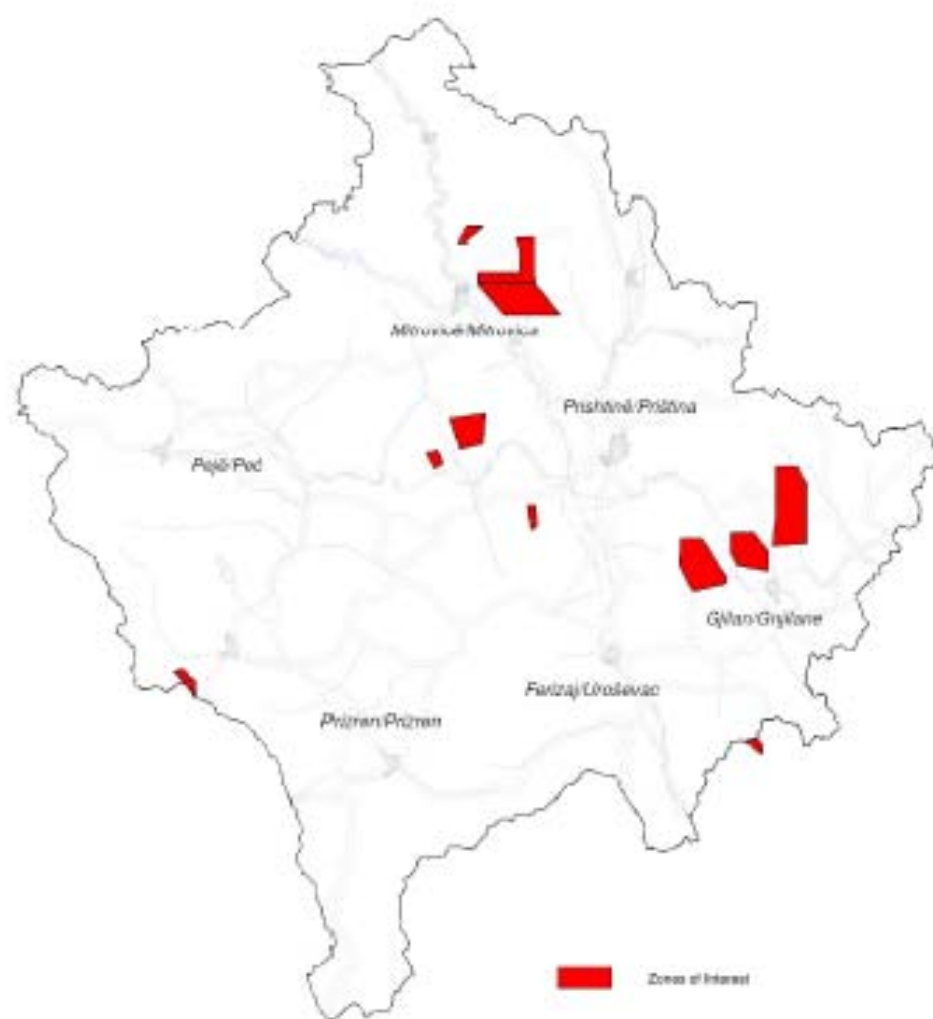
Figura 25. Hartë vështruese e zonave të interesit
