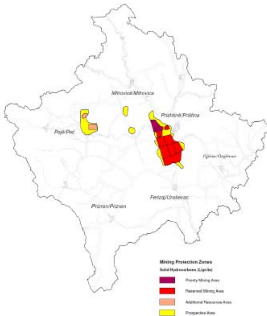
Figura 24. Hartë vështruese e zonave të mbrojtura minerare të hidrokarbureve të ngurta (linjiteve)
