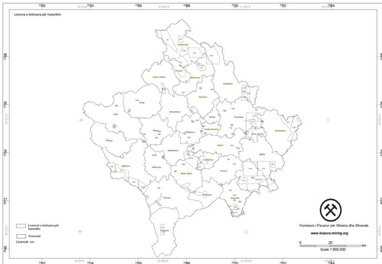
Figura 6. Harta e licencave të hulumtimit
