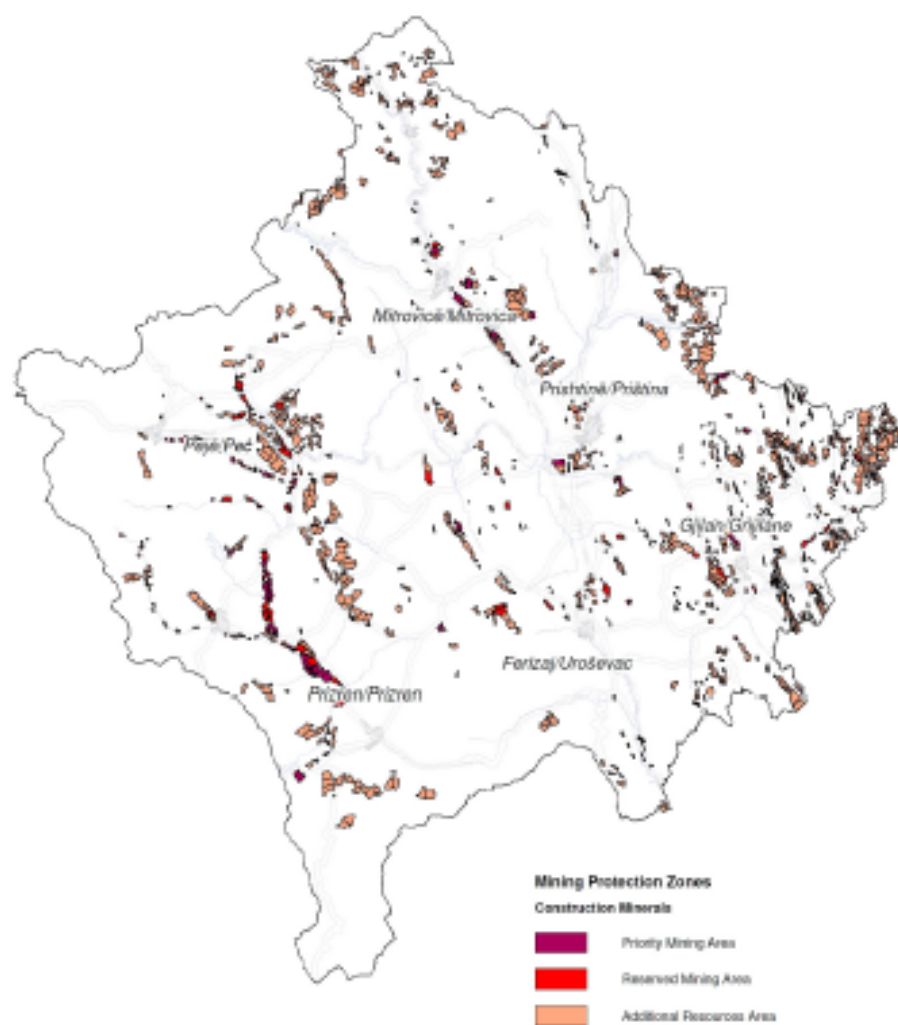
Figura 22. Hartë vështruese e zonave të mbrojtura minerare të mineraleve ndërtimore
